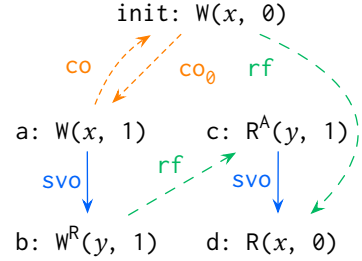
Fig. 8. Specified Visibility
