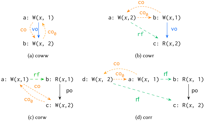
Fig. 7. Coherence
