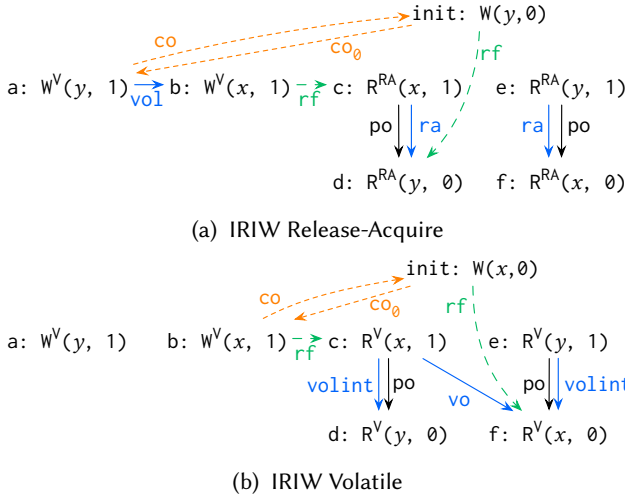
Fig. 12. IRIW Variants
