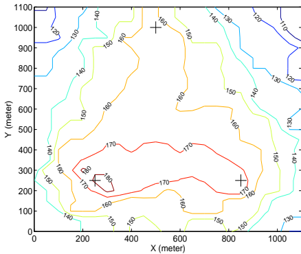
6.1: Temperature diffusion
