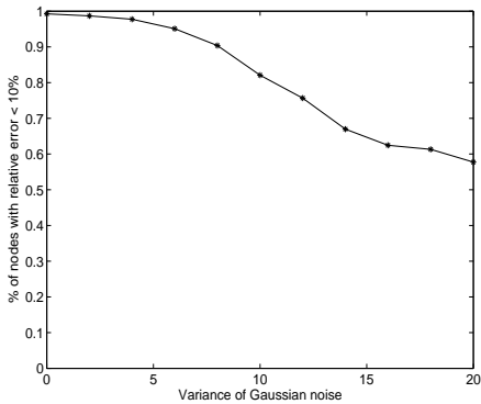
9.1: Temperature diffusion
