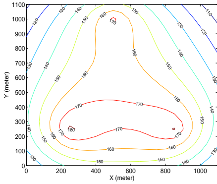
5.1: Temperature diffusion
