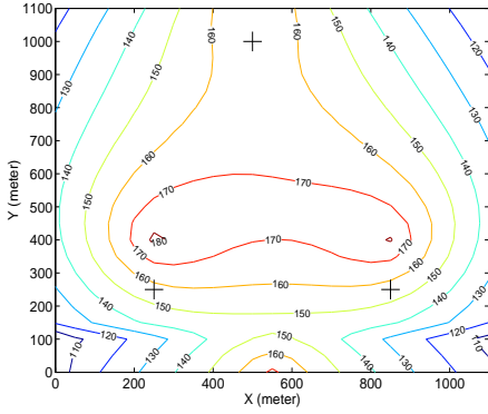
4.1: Temperature diffusion
