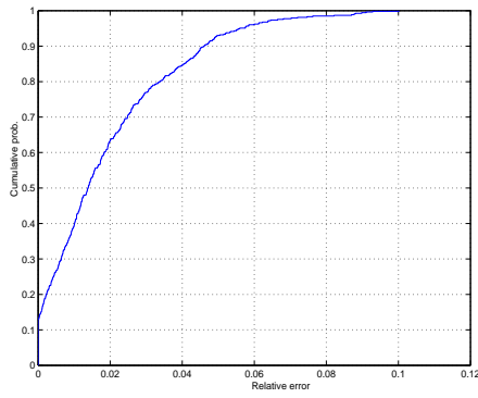
7.1: Temperature diffusion
