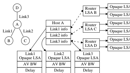
Fig. 3. Router LSAs.
